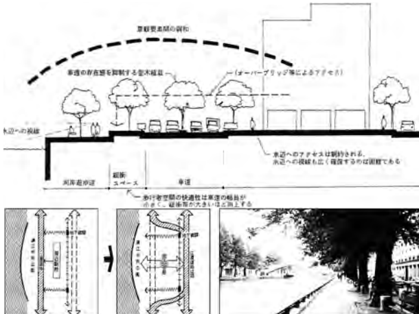
「漢江総合整備計画」で提案された沿川道路の回避 緑地による緩衝事例（パリ、サンマルタン運河）
